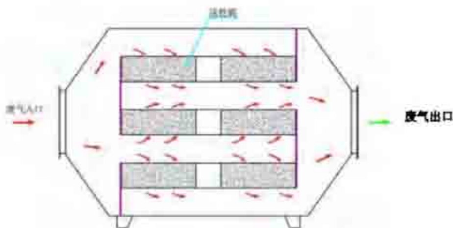
图 8-4 活性炭吸附原理示意图
