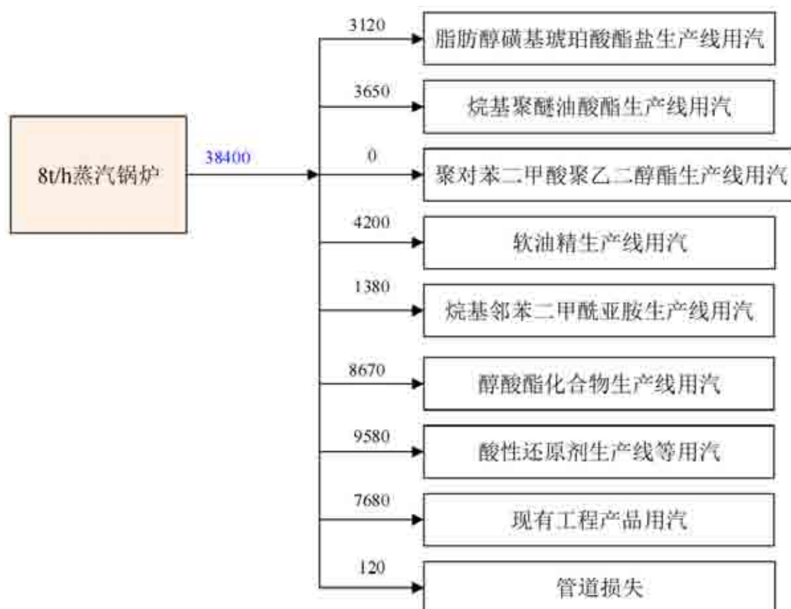
图 4-23 全厂蒸汽平衡示意图 单位：t/a
