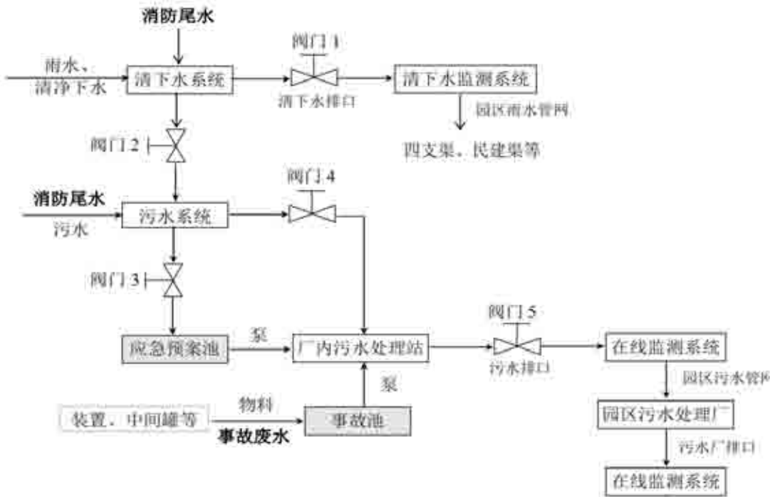
图 7-47 事故废水防范和处理流程示意图
