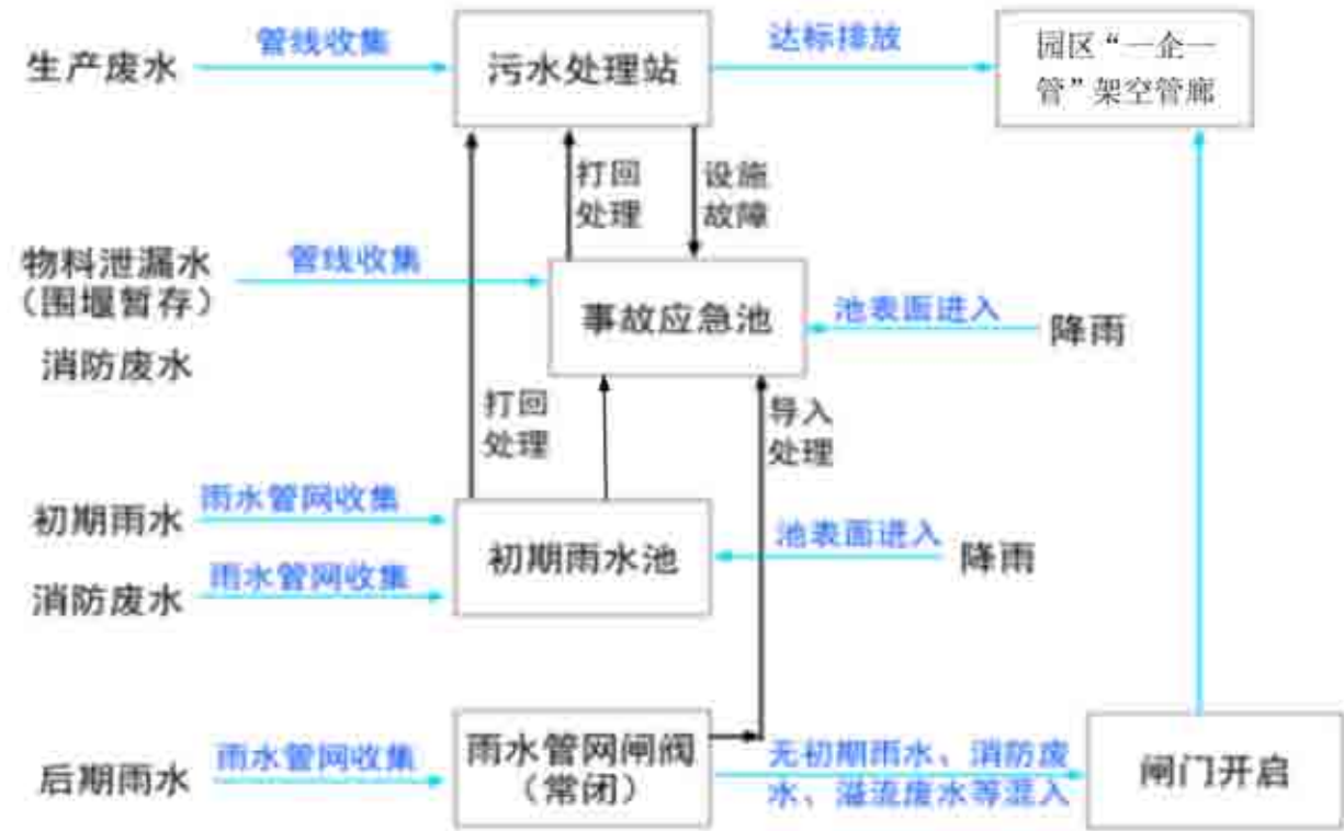
图 7-45 项目水环境风险防控体系封堵措施体系示意图
