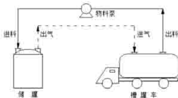
图 8-5 物料进入储罐时的无组织排放控制
