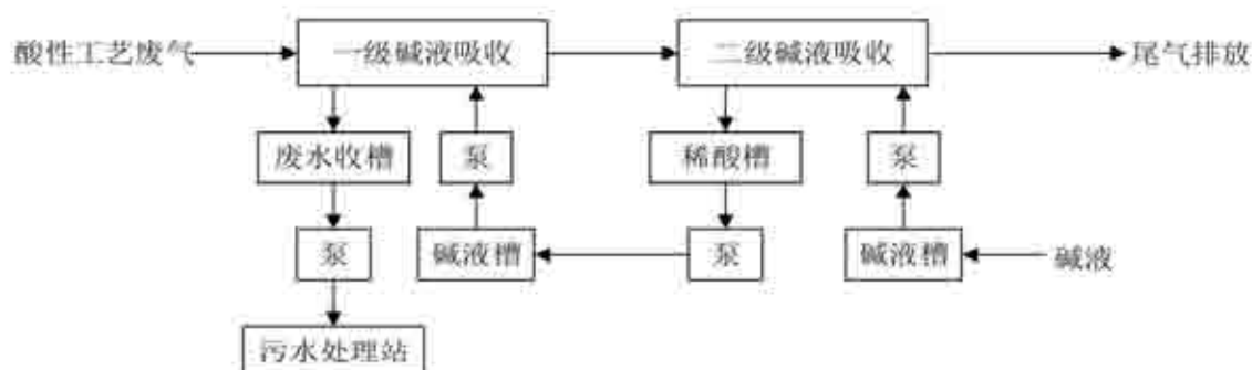
图 8-3 二级碱喷淋吸收装置工作原理
