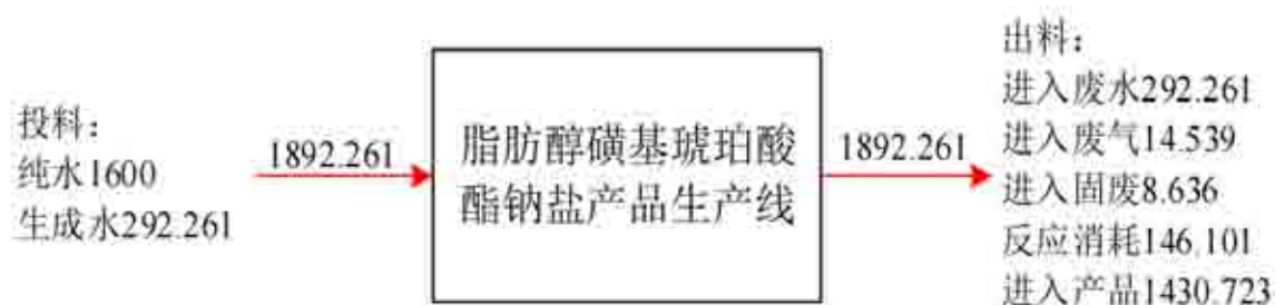
图 4-3 脂肪醇磺基琥珀酸酯钠盐产品工艺水平衡图 单位: t/a
