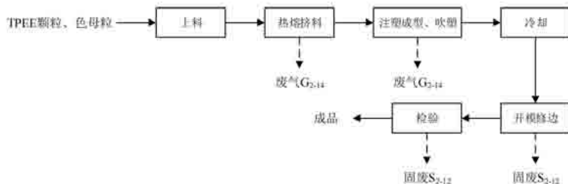
图 2-17 塑料包装桶工艺流程及产污环节图
