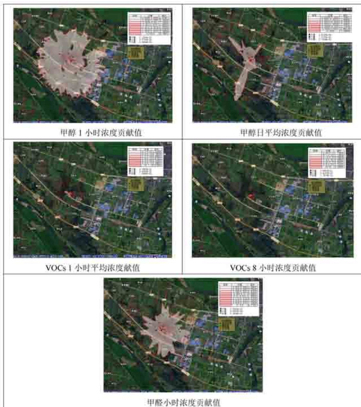
图 6-4 正常工况预测结果汇总图
