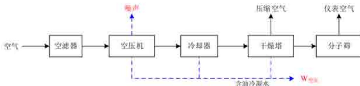
图 4-21 空气压缩站工艺流程及产污节点示意图
