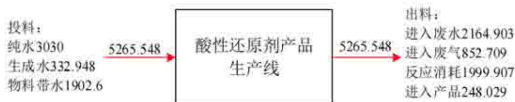
图 4-20 酸性还原剂产品工艺水平衡图 单位: m 3 /a
