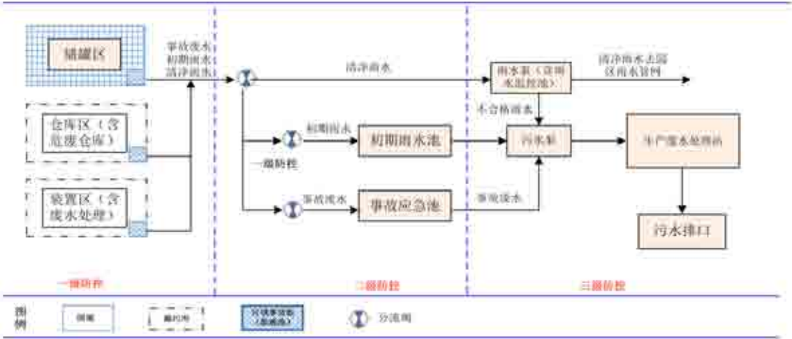
图 7-48 事故废水“三级防控”系统示意图
