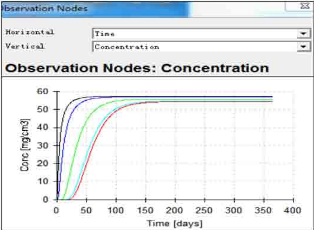
图 6-15 各观测点苯胺类污染物浓度-时间曲线图
