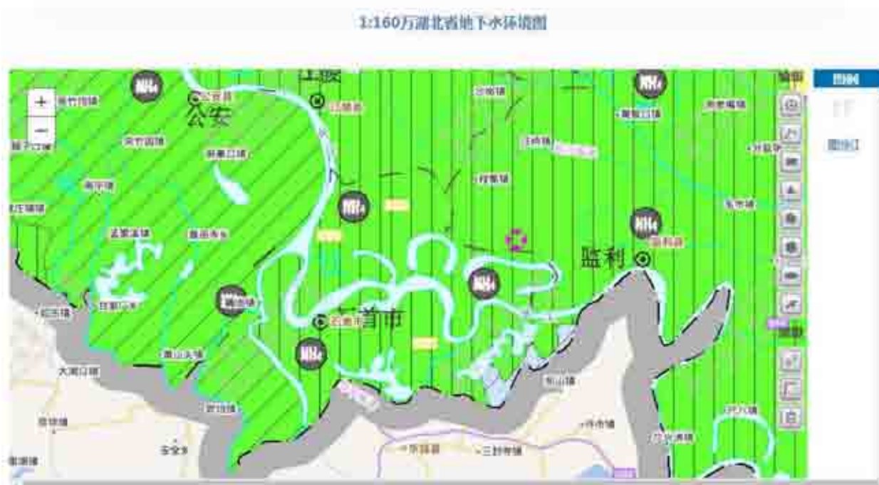
图 6-10 项目所在区域地下水环境图
