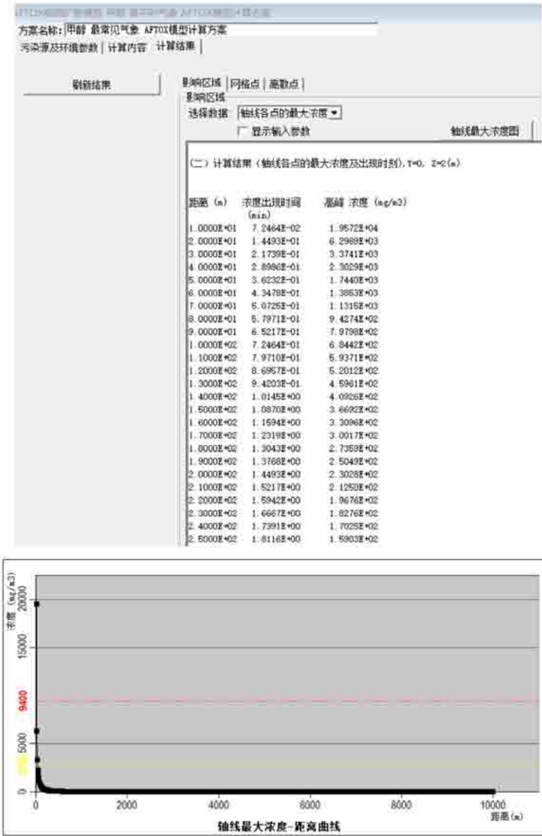
图 7-15 最常见气象条件下，下风向不同距离处，甲醇最大浓度分布图
