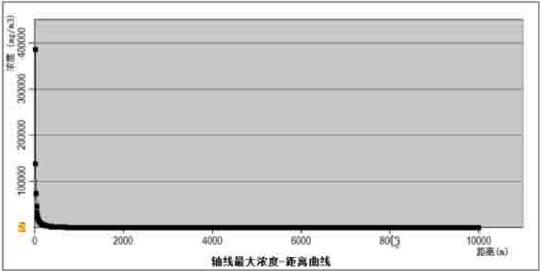
图 7-6 最不利气象条件下，下风向不同距离处，甲醛最大浓度分布图
