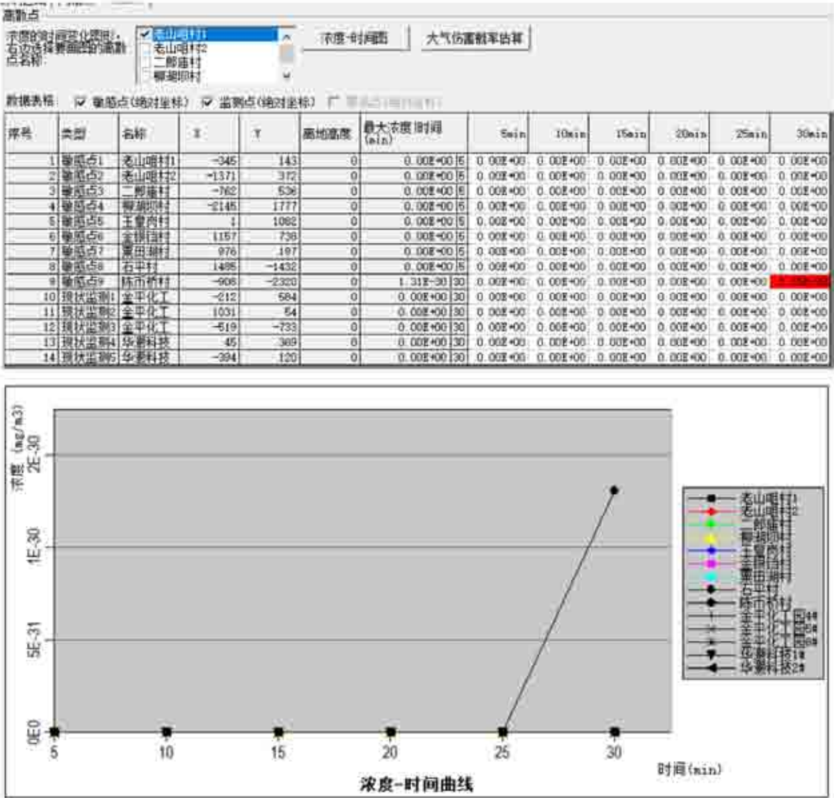
图 7-8 敏感点处甲醛浓度随时间变化图
