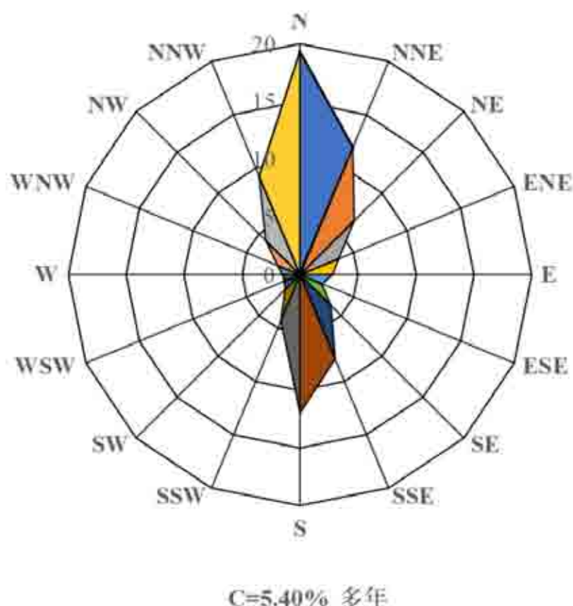
图 6-1 石首市近 20 年风向玫瑰图（静风频率 5.4%）
