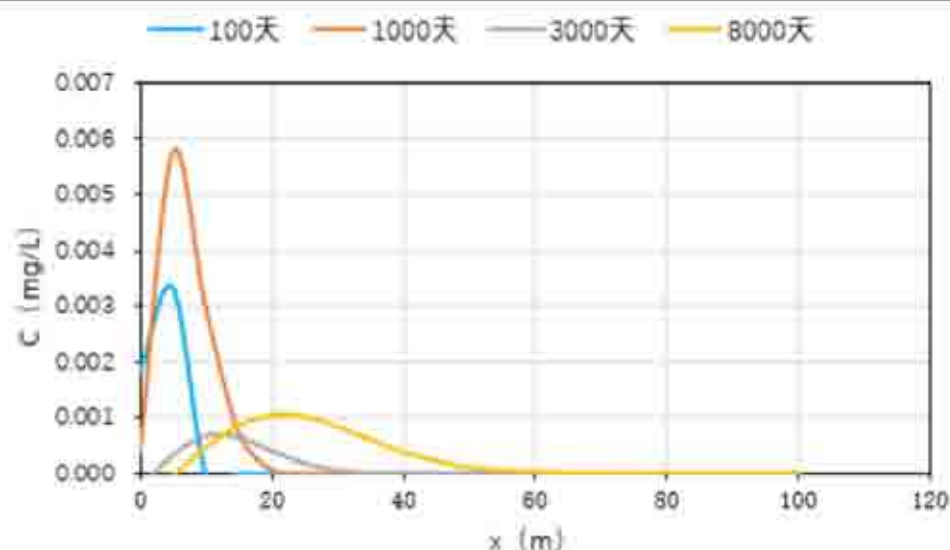
图 7-42 甲醛清洗废水泄漏污染物地下运移浓度变化
