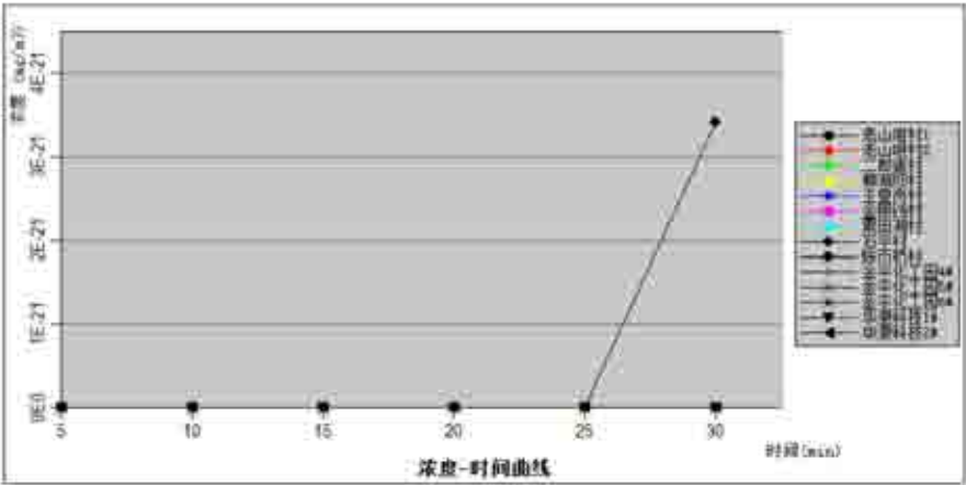
图 7-26 敏感点处异丙醇浓度随时间变化图
