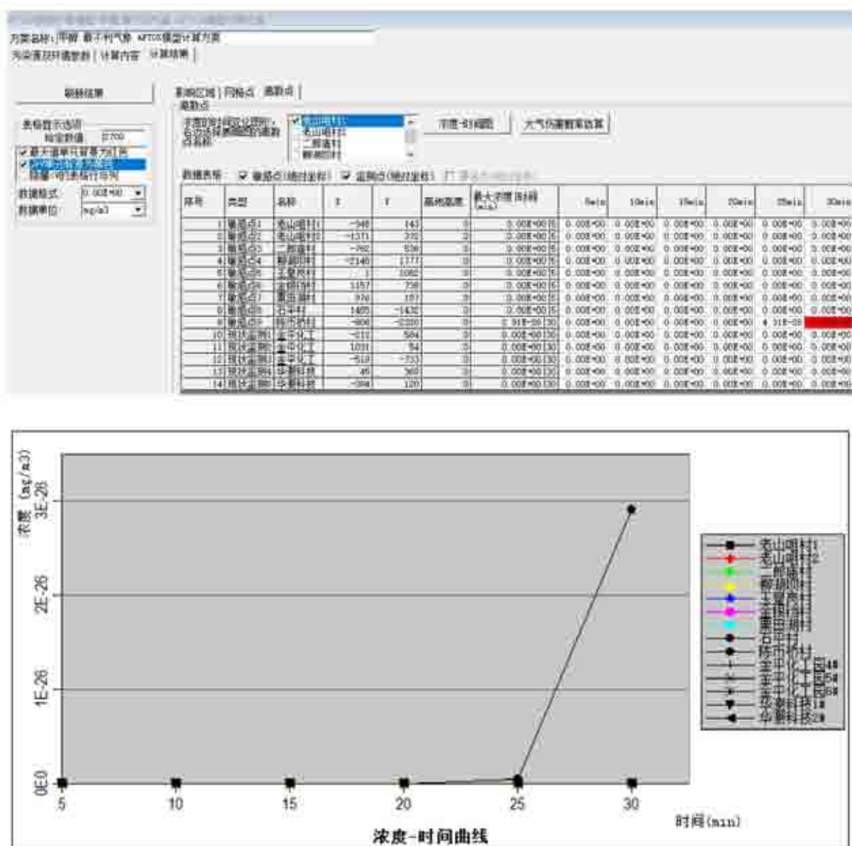
图 7-14 敏感点处甲醇浓度随时间变化图
