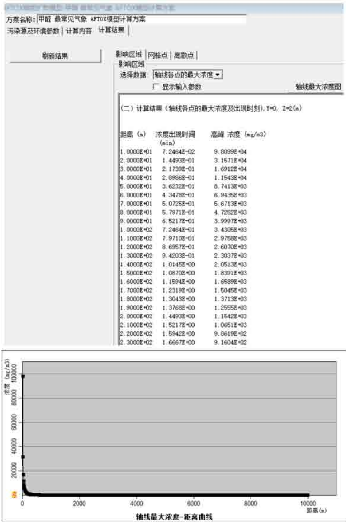
图 7-9 最常见气象条件下，下风向不同距离处，甲醛最大浓度分布图
