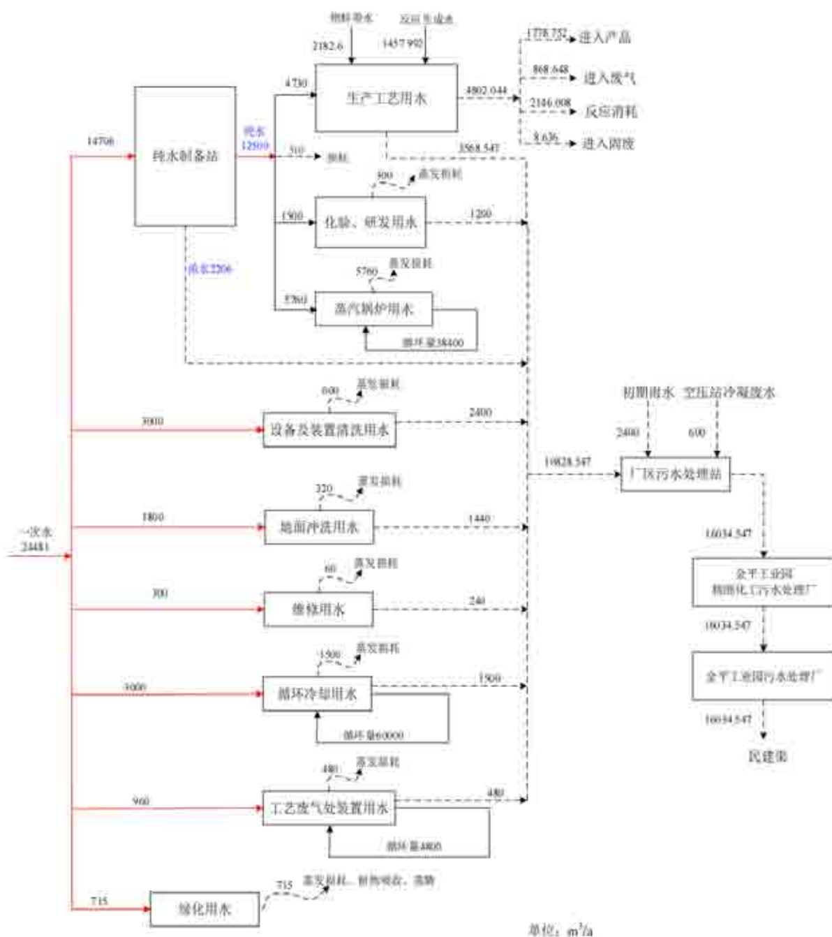
图 4-22 项目水平衡分析图 单位: \text{m}^3/\text{a}
