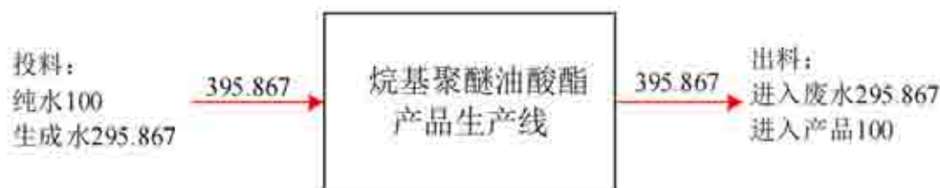
图 4-15 烷基聚醚油酸酯产品工艺水平衡图 单位：m³/a
