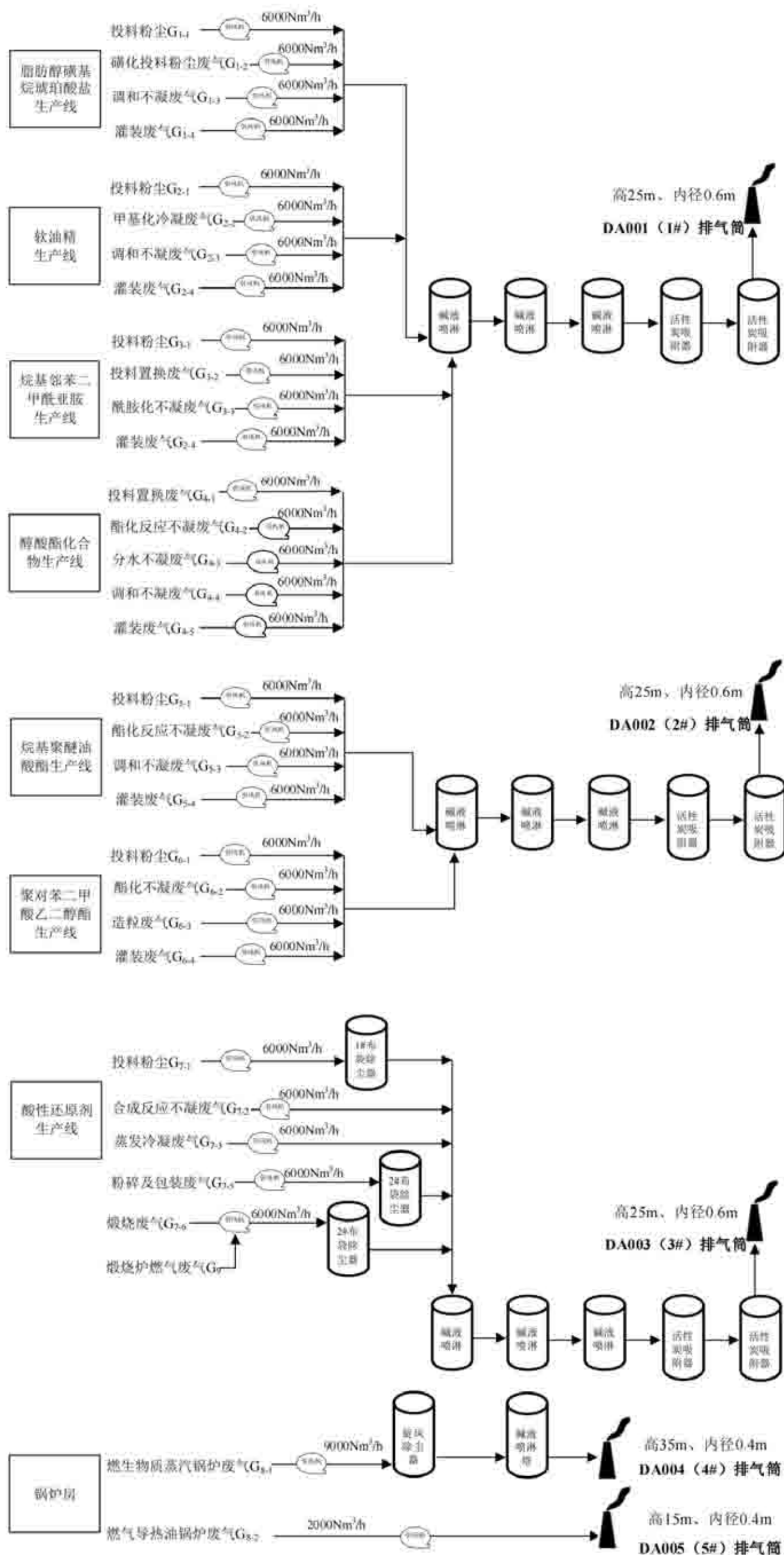
图 8-1 项目废气治理措施示意图
