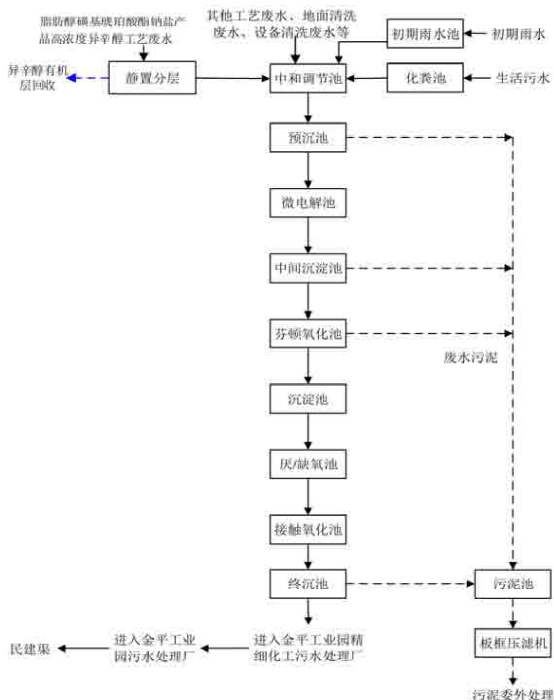
图 8-6 项目废水处理站工艺流程图
