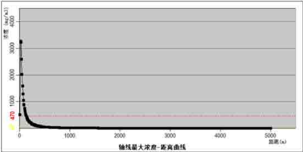
图 7-21 最常见气象条件下，下风向不同距离处，甲酸最大浓度分布图
