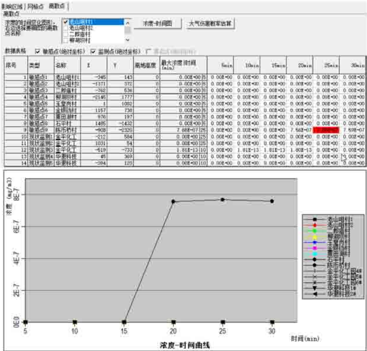
图 7-17 敏感点处甲醇浓度随时间变化图
