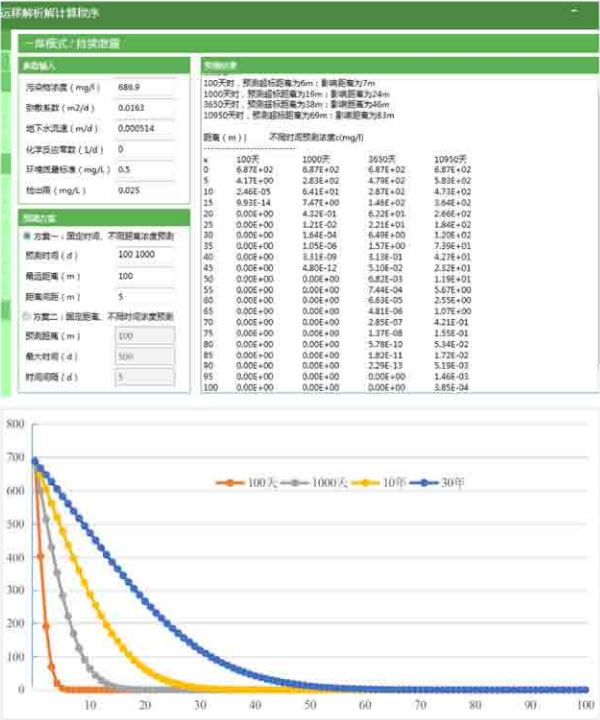
图 6-13 连续泄漏氨氮污染扩散距离图
