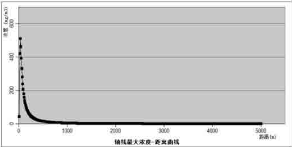
图 7-27 最常见气象条件下，下风向不同距离处，异丙醇最大浓度分布图
