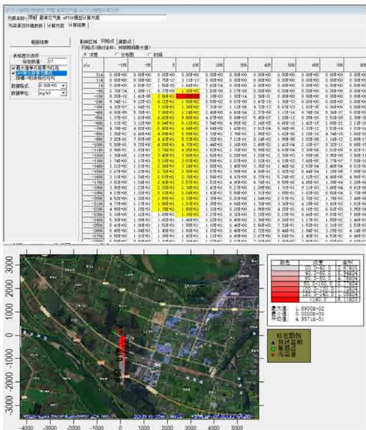
图 7-10 最常见气象条件下, 甲醛各网格点浓度分布图
