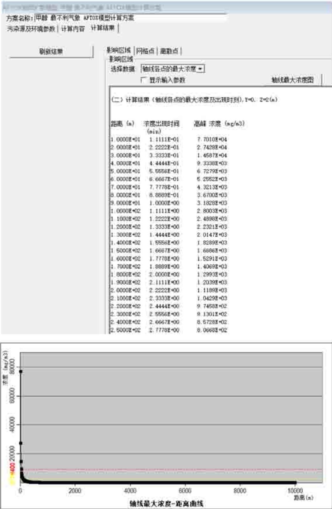
图 7-12 最不利气象条件下，下风向不同距离处，甲醇最大浓度分布图
