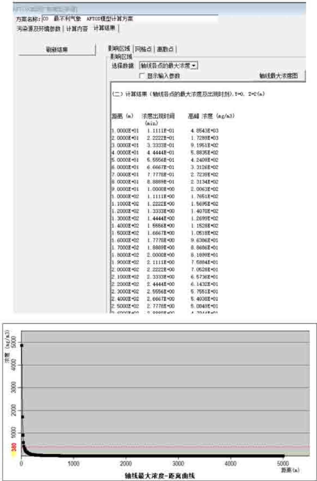
图 7-36 最不利气象条件下，下风向不同距离处，CO 最大浓度分布图
