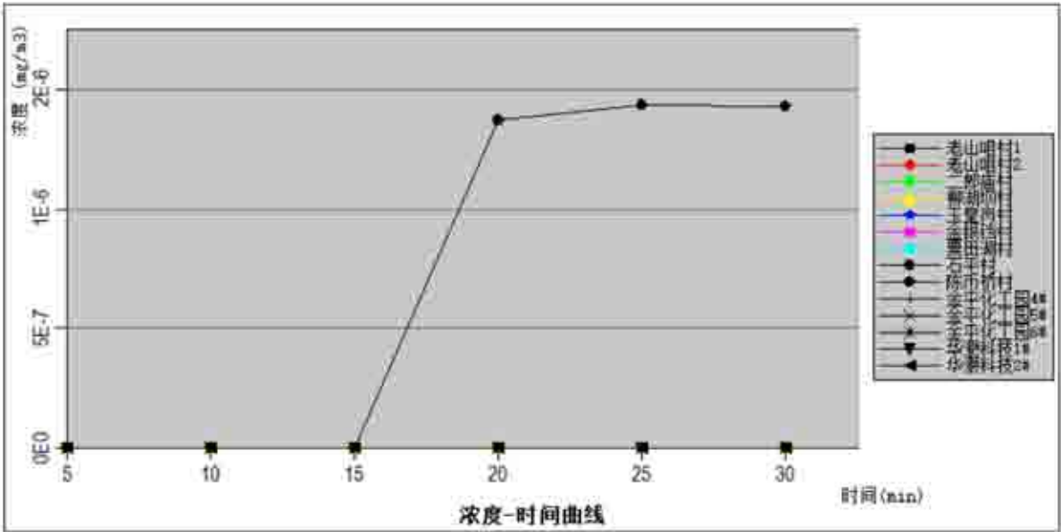
图 7-35 敏感点处硫酸二甲酯浓度随时间变化图
