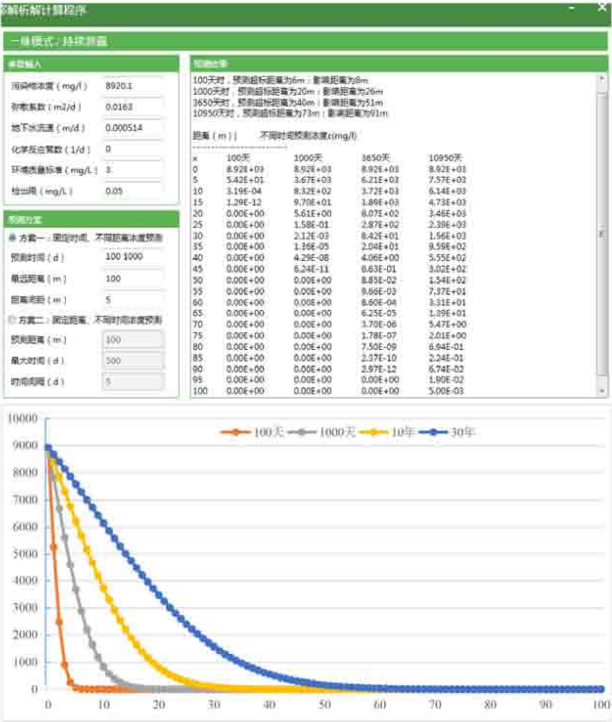
图 6-12 连续泄漏 COD 污染扩散距离图
