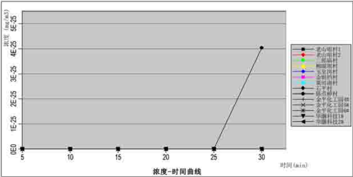
图 7-32 敏感点处硫酸二甲酯浓度随时间变化图
