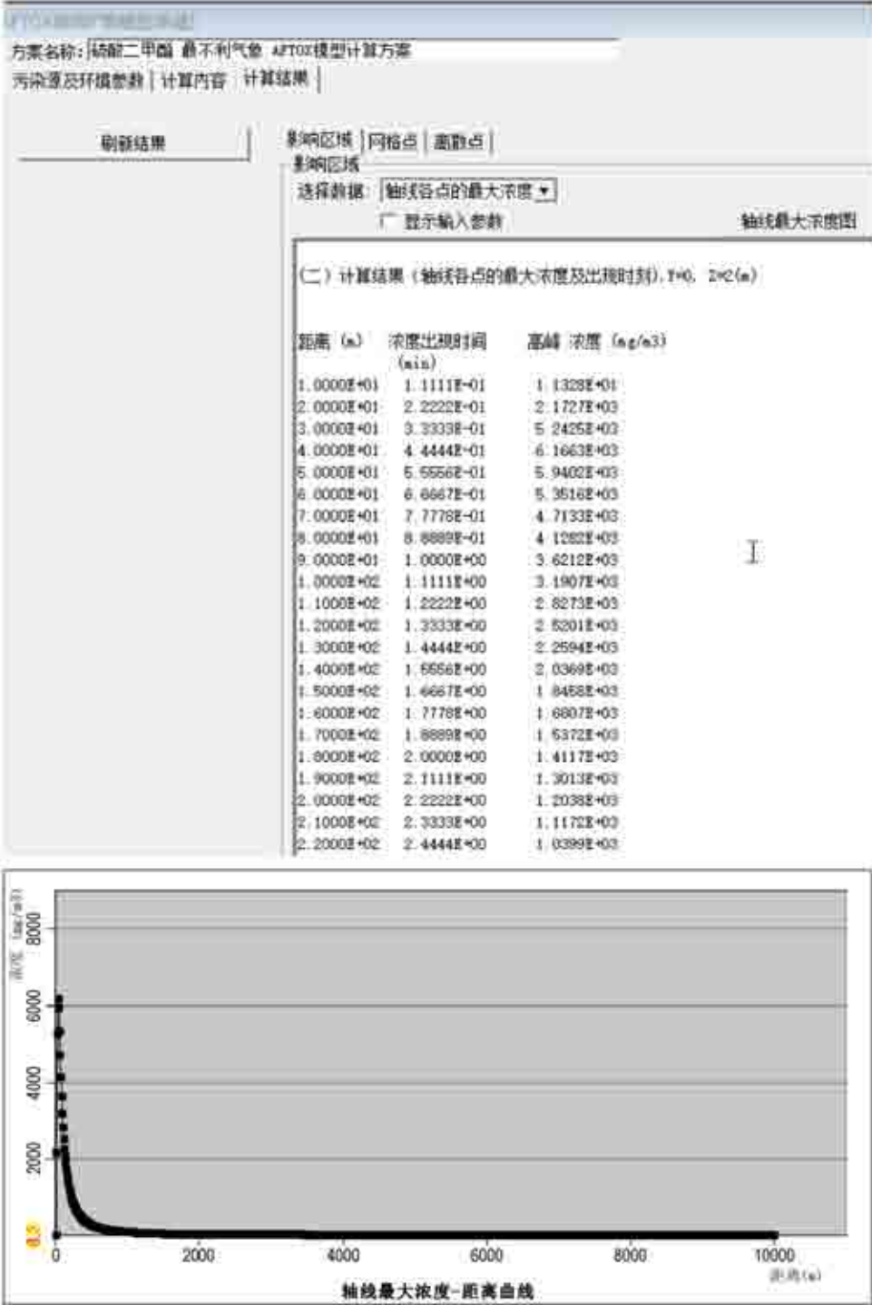
图 7-30 最不利气象条件下, 下风向不同距离处, 硫酸二甲酯最大浓度分布图
