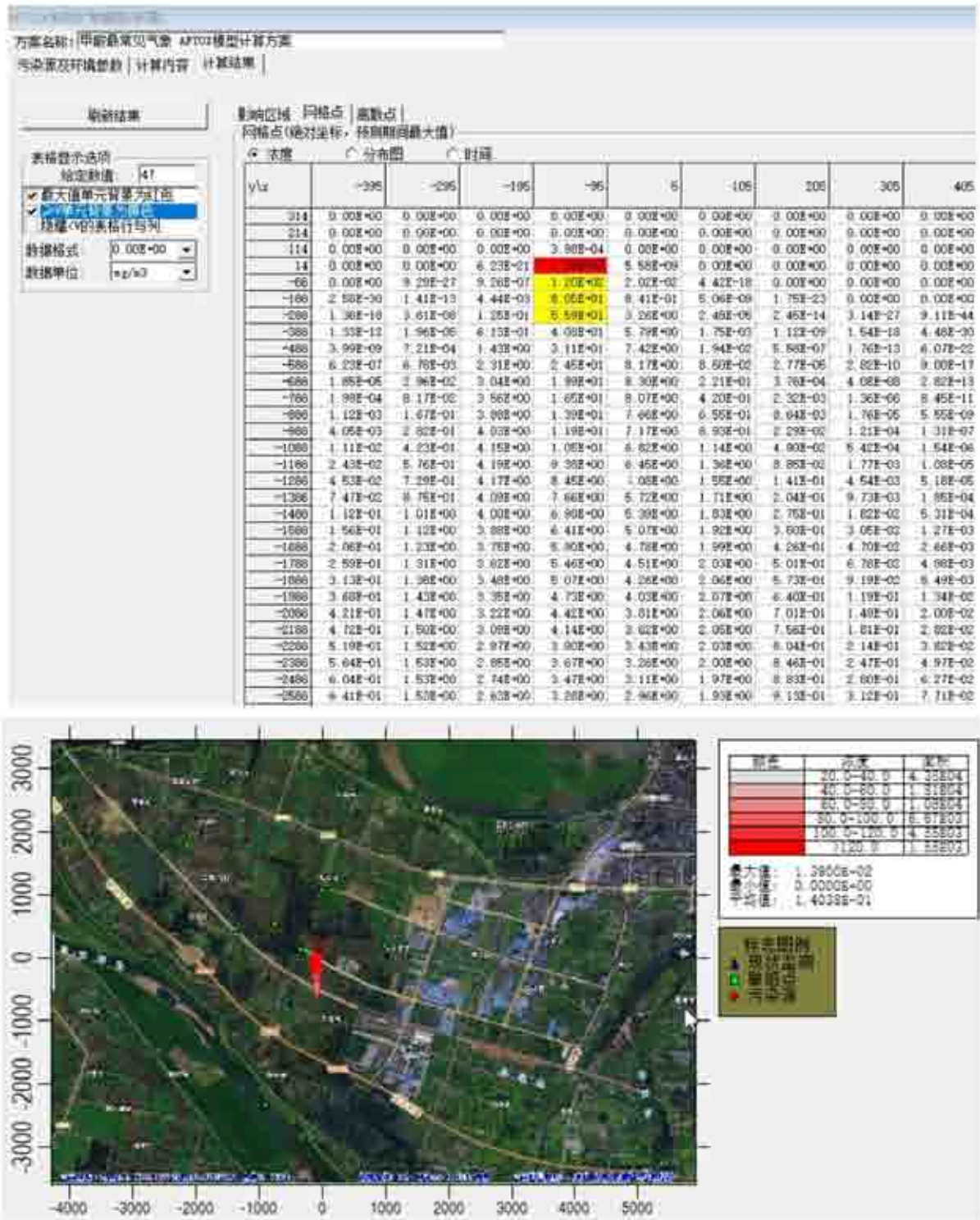
图 7-22 最常见气象条件下，甲酸各网格点浓度分布图
