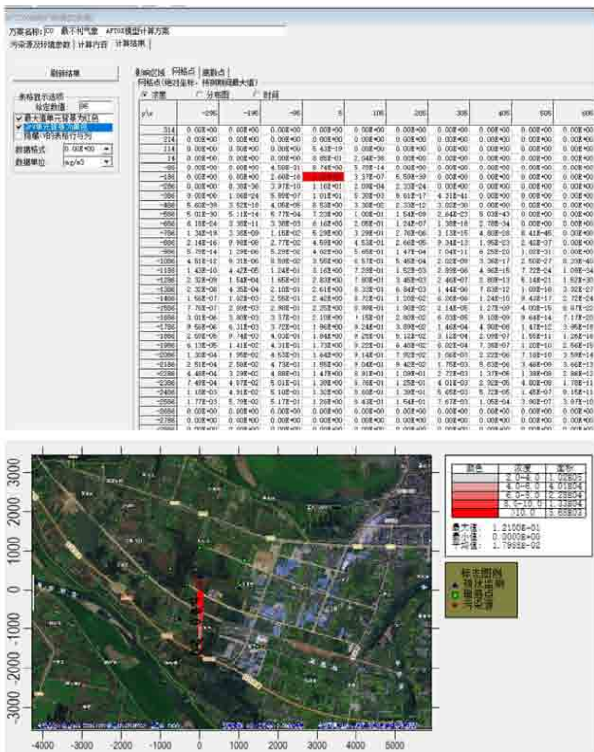
图 7-37 最不利气象条件下, CO 各网格点浓度分布图
