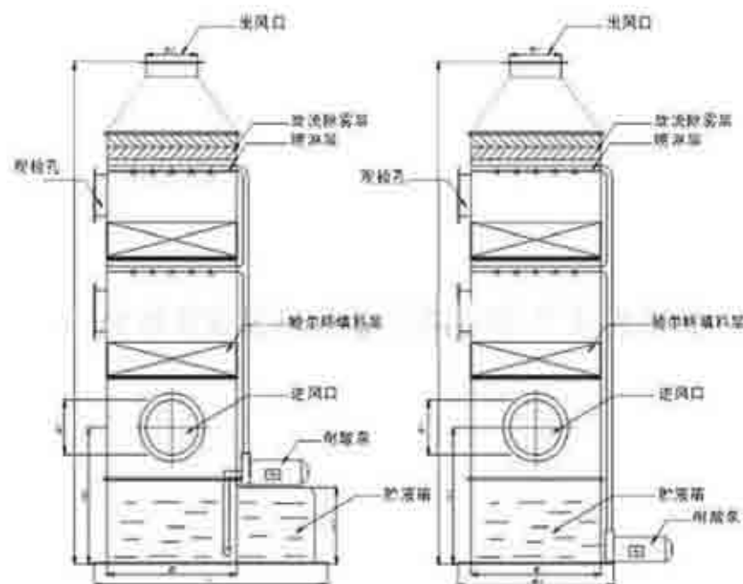
图 8-2 喷淋塔处理工艺示意图
